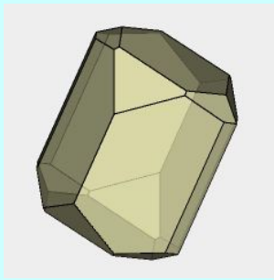
typische Kristallformen
