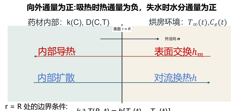
(c) 药材表面热湿交换边界示意
