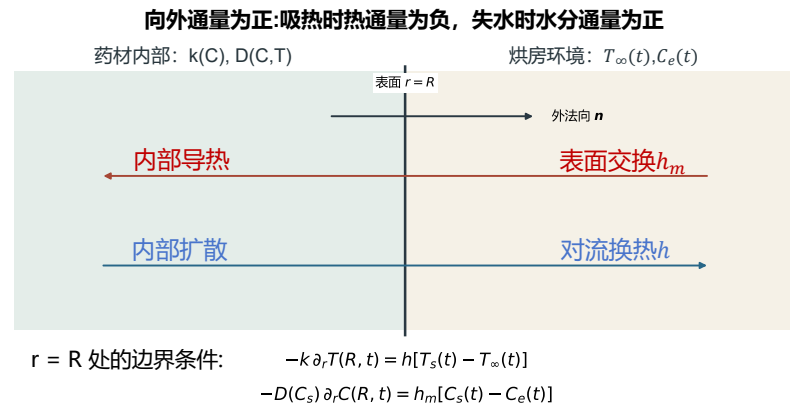
(c) 药材表面热湿交换边界示意
