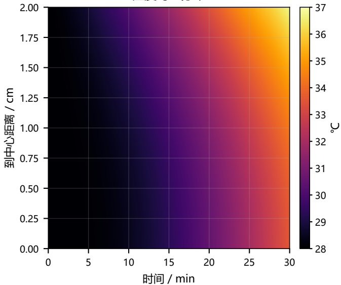
温度时空分布
