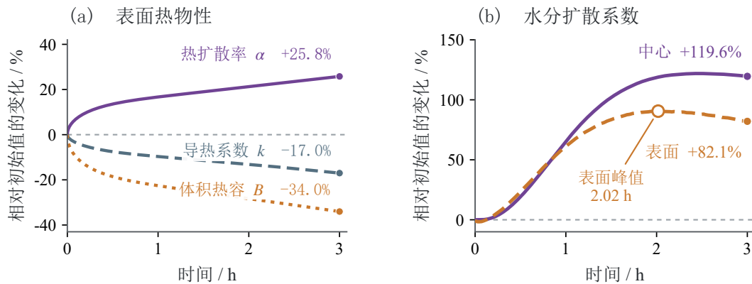
图 6: 烘干过程中热物性和水分扩散系数的变化
