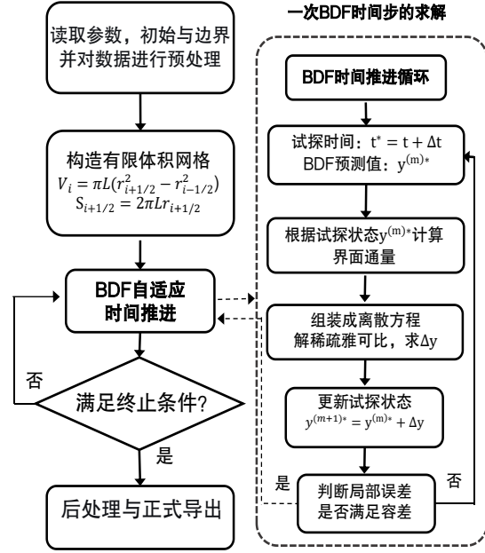
图 3: 预热阶段温湿分布的计算流程
