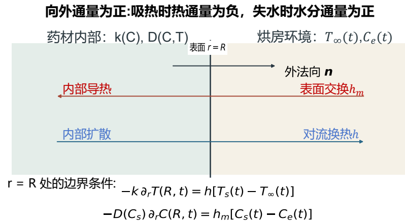
(c) 药材表面热湿交换边界示意
