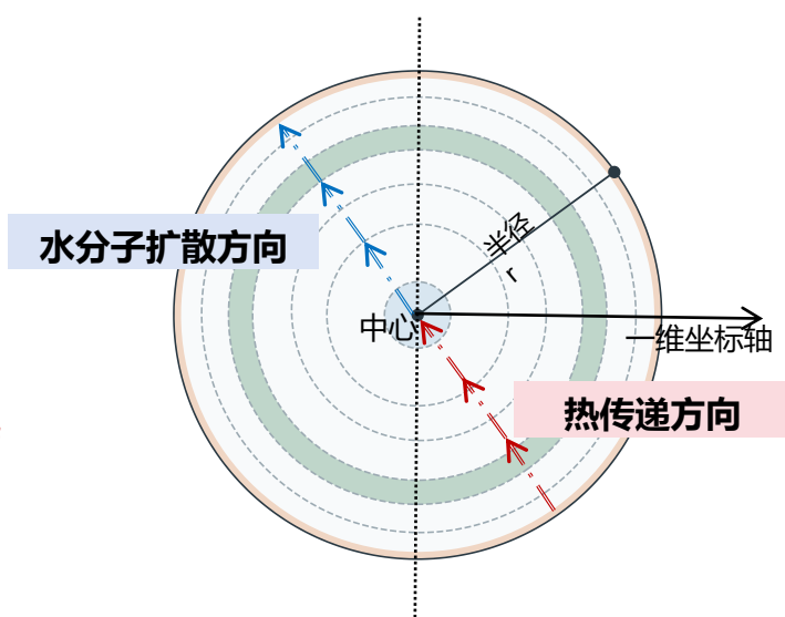
(b) 环形控制体积【药材截面】
