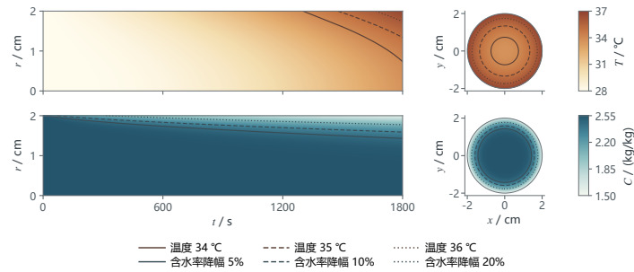
图 4: 预热阶段温湿时空分布与末态中截面；圆形截面由径向解作轴对称映射得到
