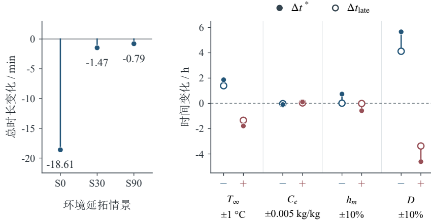
图 11: 环境与传质参数变化对总时长和末期耗时的影响
