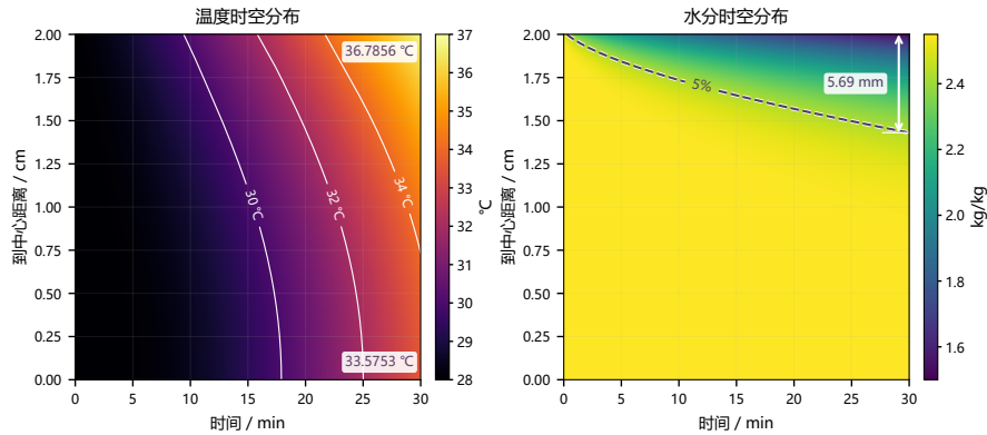
图 4: 预热阶段温湿时空分布
