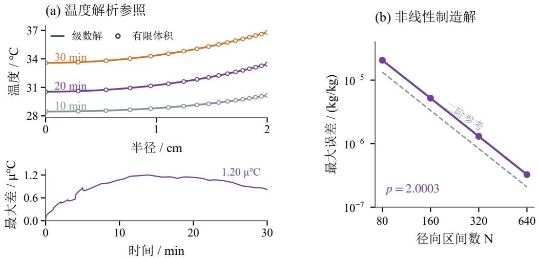
图 5: 第一问的独立参照检验：温度级数解与非线性水分制造解
