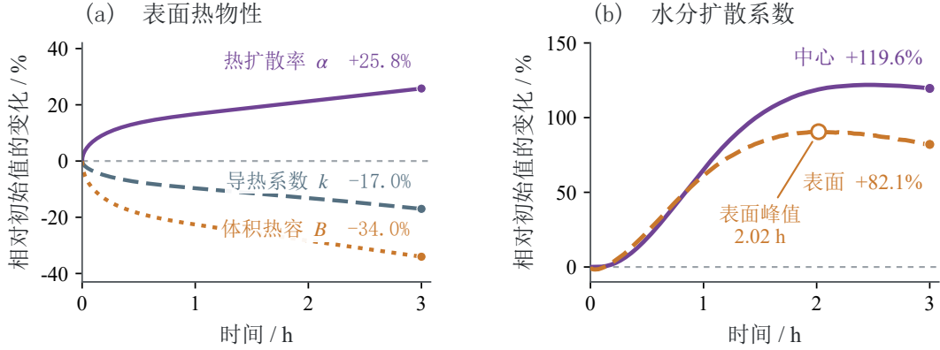
图 6: 烘干过程中热物性和水分扩散系数的变化
