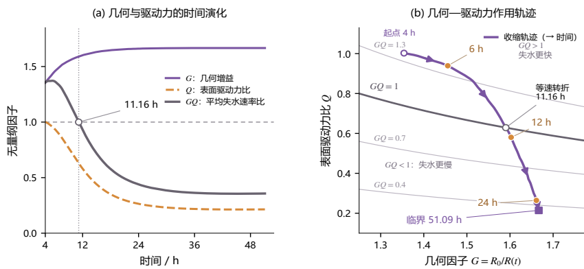
图 14: 几何变化与表面驱动力对平均含水率下降速度的共同作用
