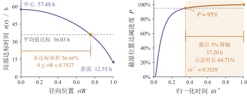
图 9: 各位置的达标次序与最湿位置的达阈进度
