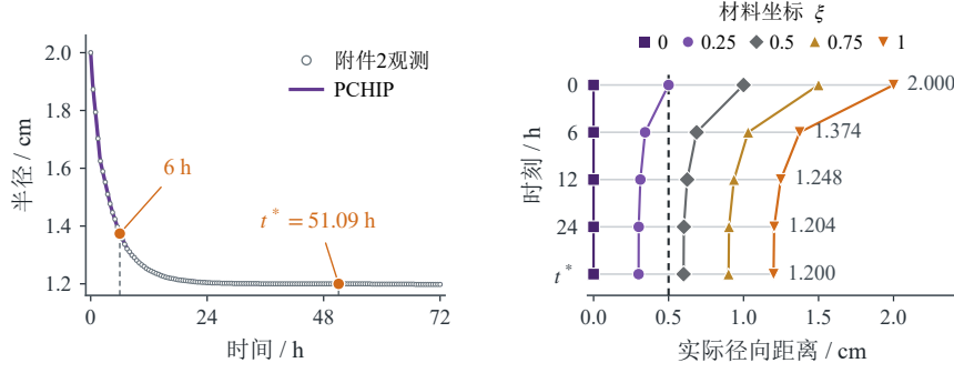
图 12: 实测半径变化及收缩过程中材料层的位置
