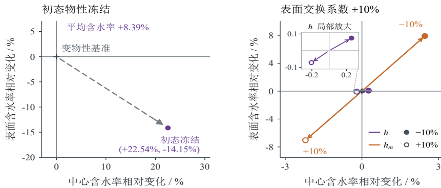
图 7: 初态物性冻结及表面交换系数扰动对含水率的影响
