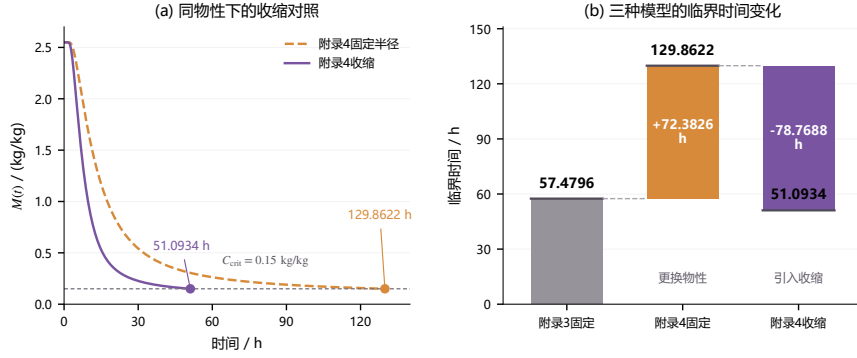
图 13: 同物性下的收缩对照及三种模型的临界时间比较
