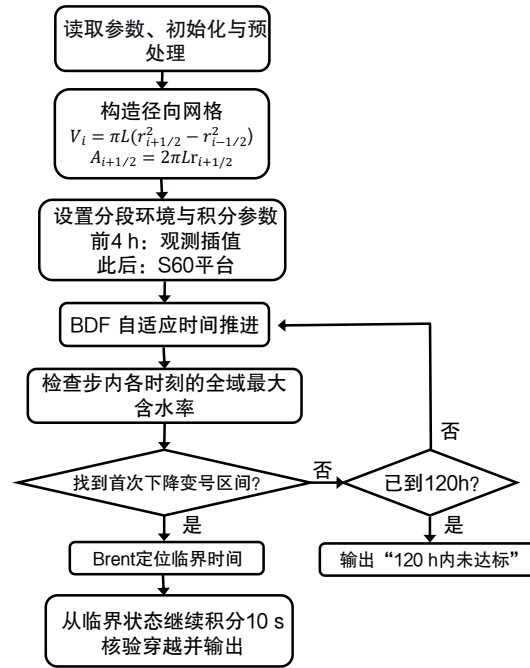
图 8: 全域首次达标时间的计算流程
