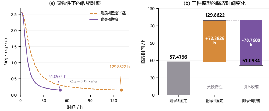
图 11: 同物性下的收缩对照及三种模型的临界时间比较
