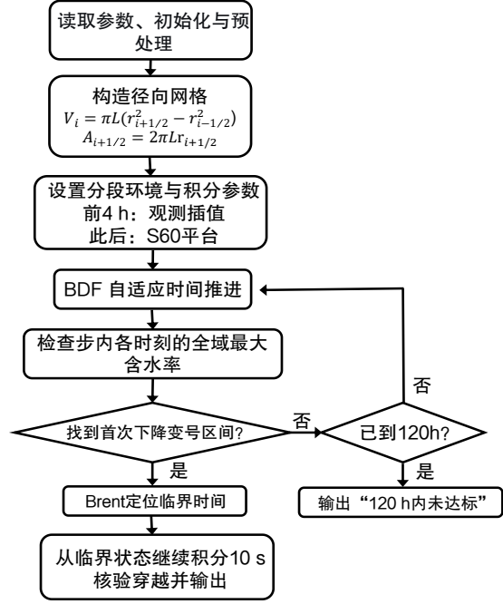
图 7: 全域首次达标时间的计算流程
