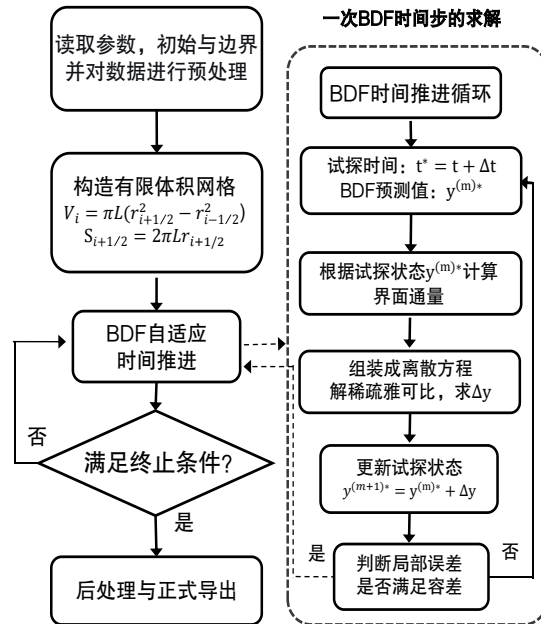
图 3: 预热阶段温湿分布的计算流程
