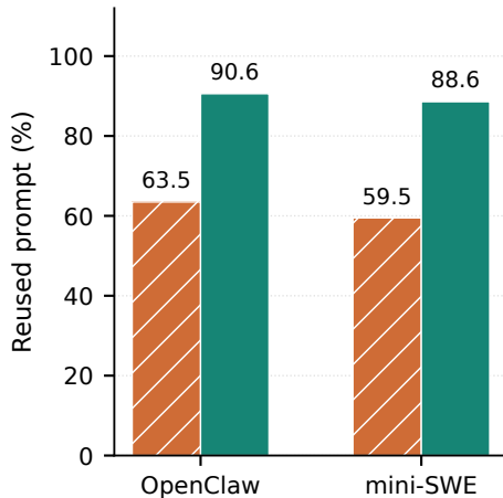
(b) Prefix reuse
