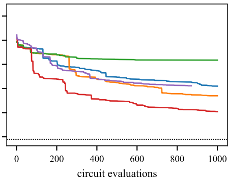
COBYLA
