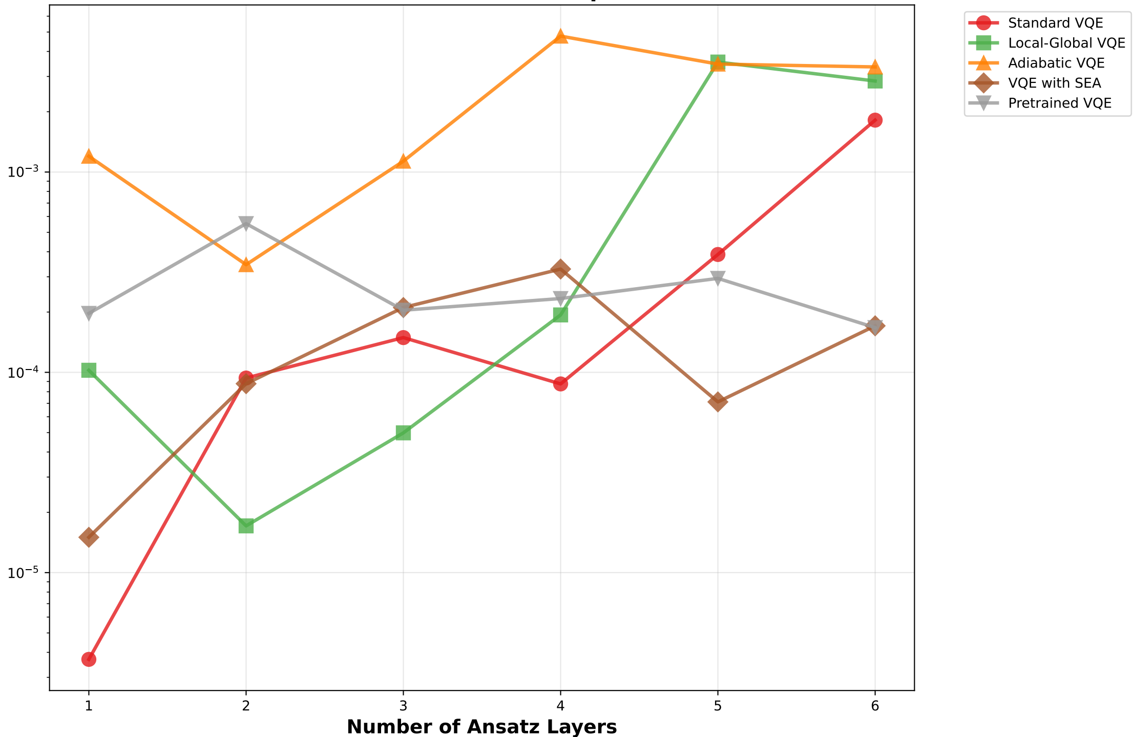
Gradient Variance vs Ansatz Depth (6 Qubits)
