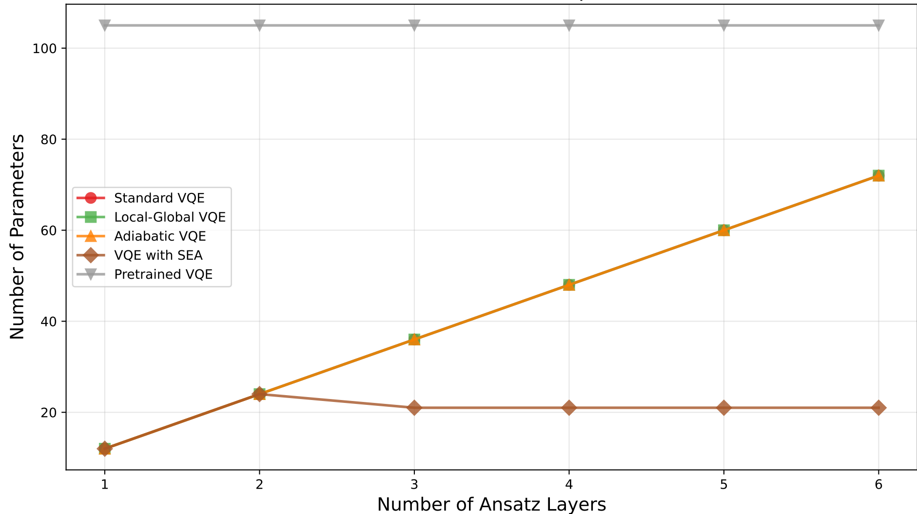
Parameter Count vs Ansatz Depth (6 Qubits)
