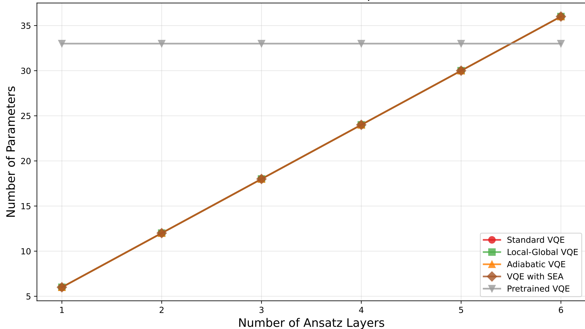
Parameter Count vs Ansatz Depth (3 Qubits)
