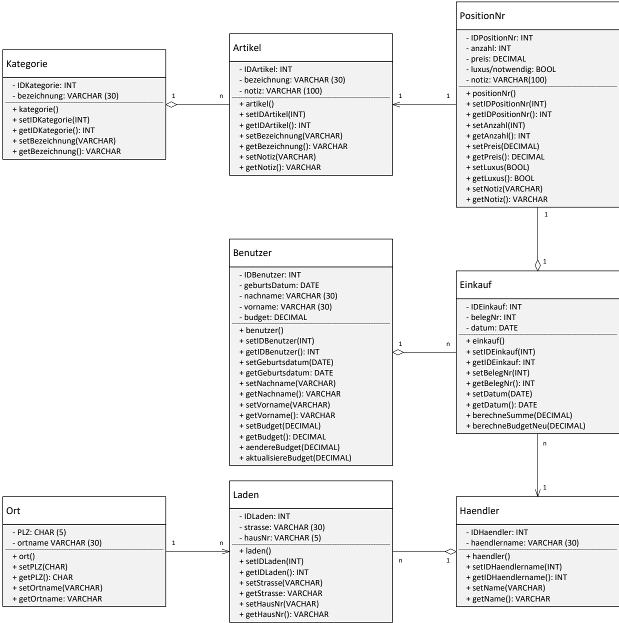
Klassendiagramm Objektorientierte Designansicht: Haushaltsbuch, Version 06, 2025-08-13
