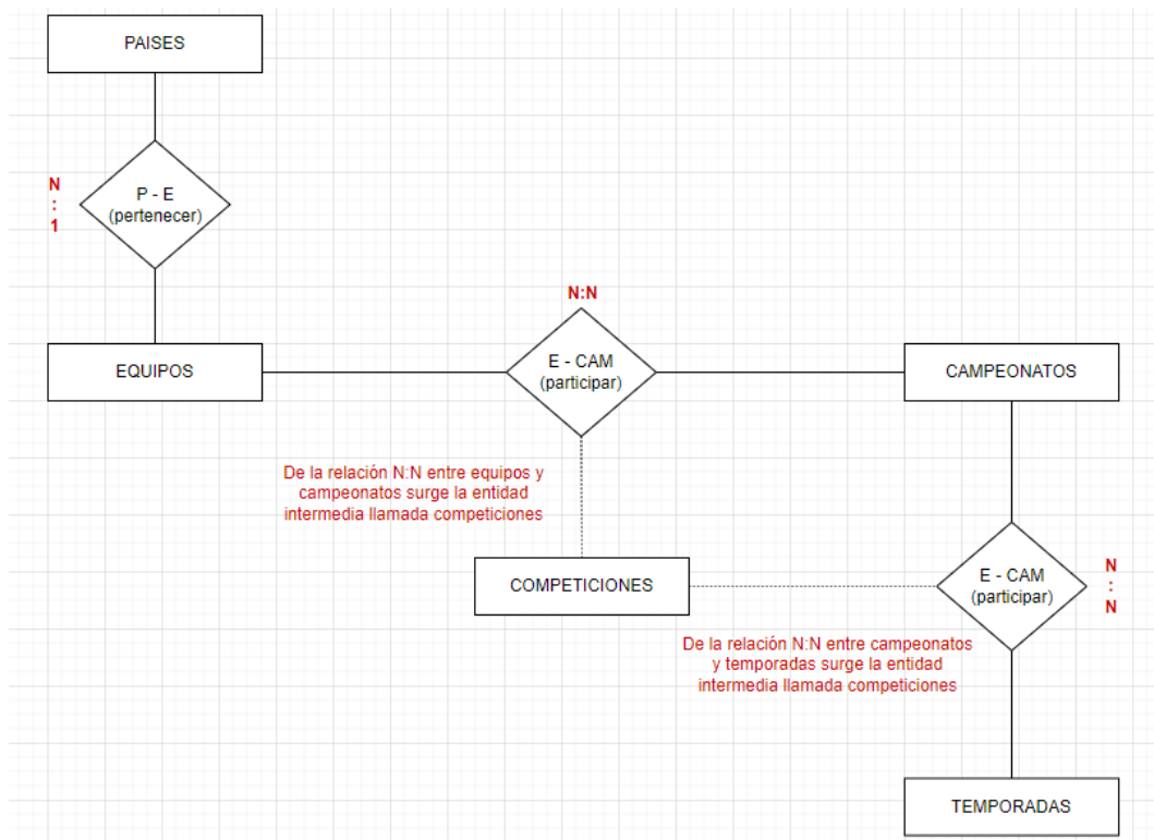
Imagen de un diagrama entidad-relación
