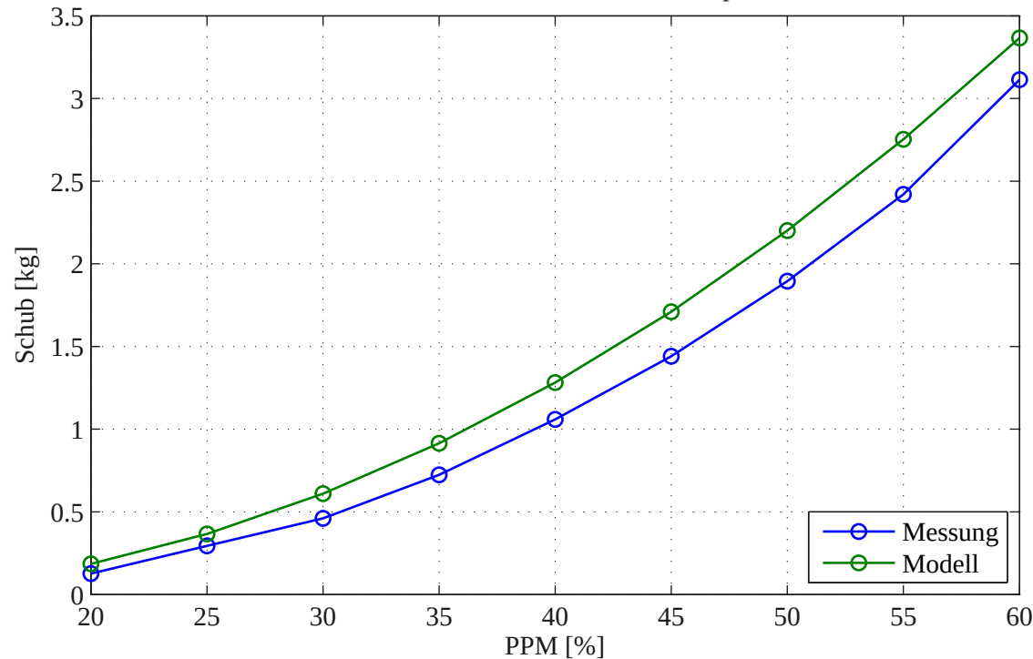
Statische Kennlinie Closed-Loop
