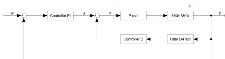
Abbildung 3: Gyro Control Loop
