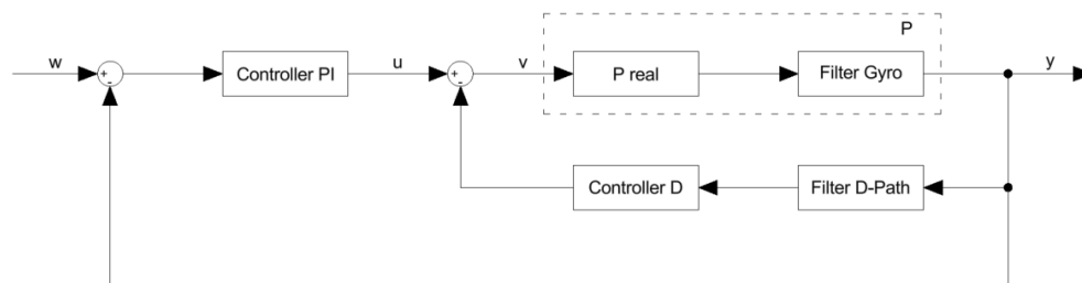
Abbildung 3: Gyro Control Loop
