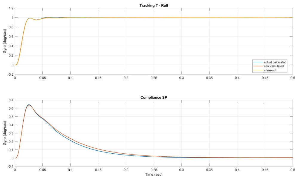
Abbildung 15: Step Response
