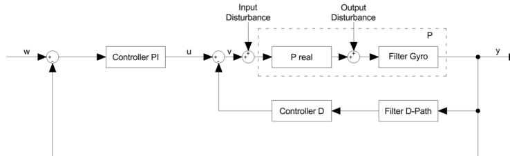
Abbildung 3: Gyro Control Loop
