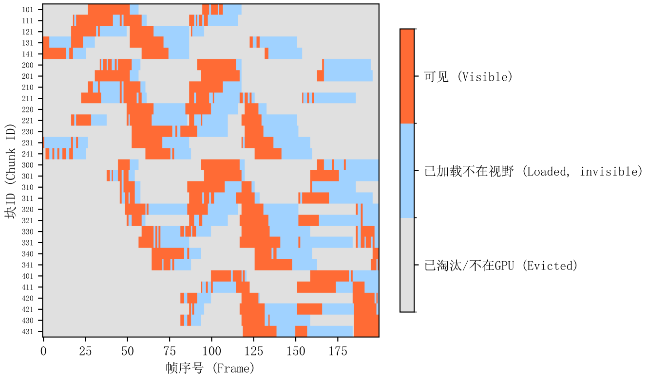
高频访问块的生命周期热力图 (Chunk Access Timeline)
