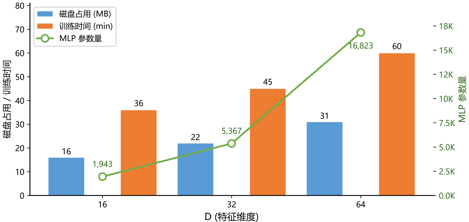
不同特征维度 D 的存储与计算开销 (KITTI/seq05, K = 5)
