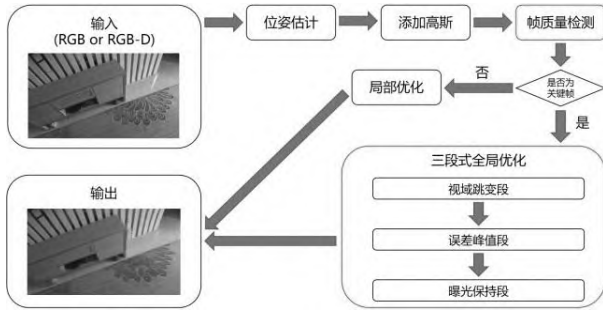
图 1 ReRTG-SLAM 方法概览。
