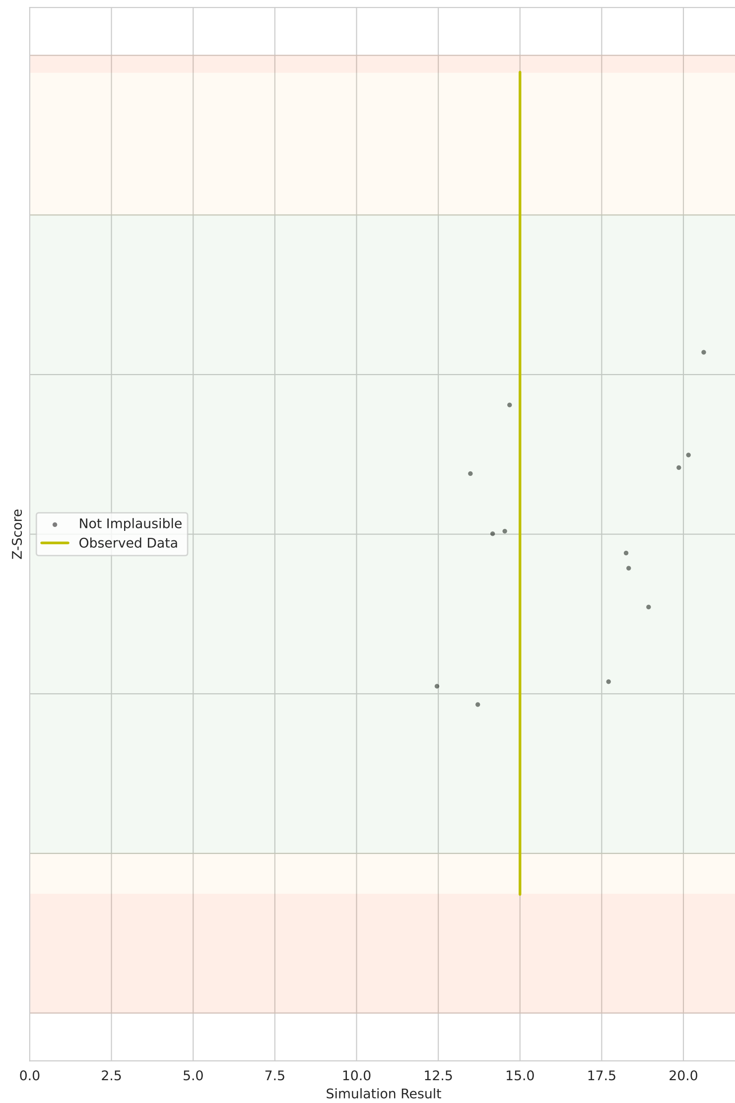
Test
