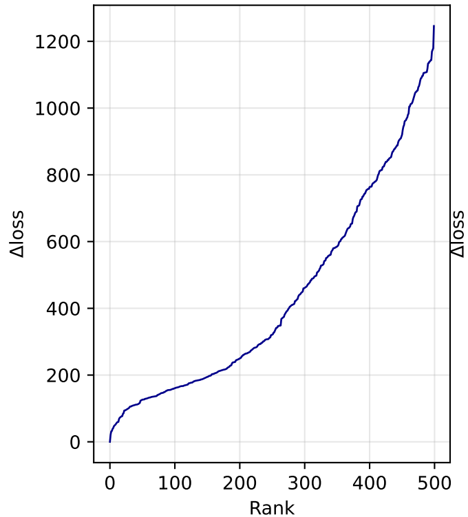
Δloss Rank
