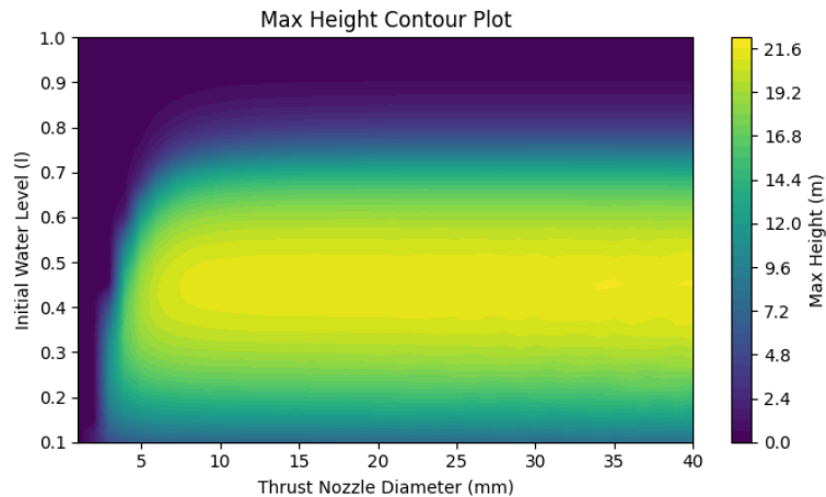
Abb. 5: Maximale Höhe der Rakete in Abhängigkeit von Wasserfüllstand und Düsendurchmesser. ( \Delta t = 0,2 \text{ ms} )
