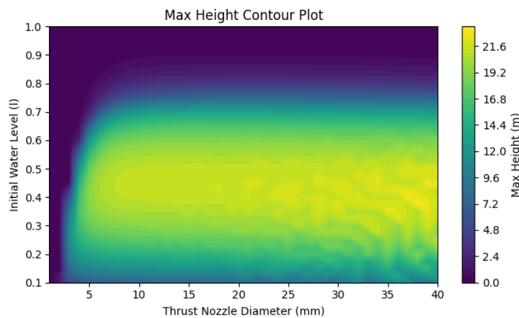
Abb. 4: Maximale Höhe der Rakete in Abhängigkeit von Wasserfüllstand und Düsendurchmesser. ( \Delta t = 1 ms)
