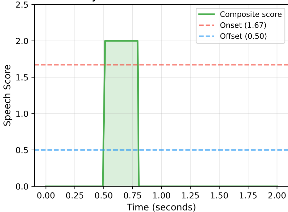
Hysteresis VAD State Machine
