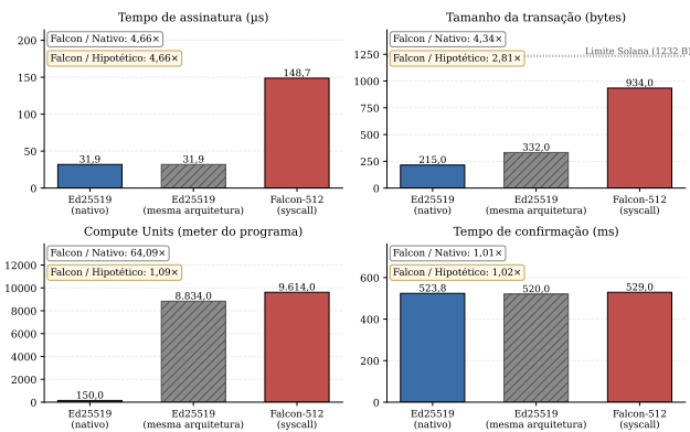
Fig. 1. Comparação entre Ed25519 nativo, Ed25519 sob mesma arquitetura (hipotético) e Falcon-512 via syscall para N = 10.000 transações. Cada painel apresenta o fator de overhead associado.
