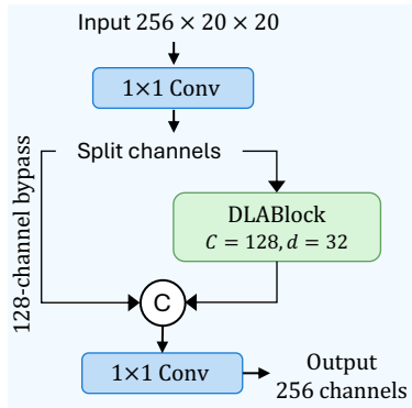
(a) C2DLA module
