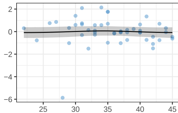
RVB
