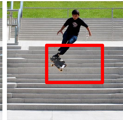
SD3
