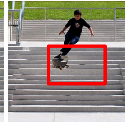
SD3
