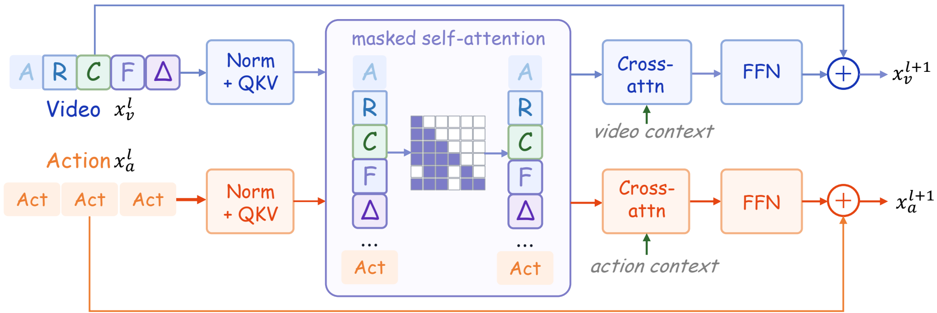
(b) WORLD-ACTION MoT LAYER
