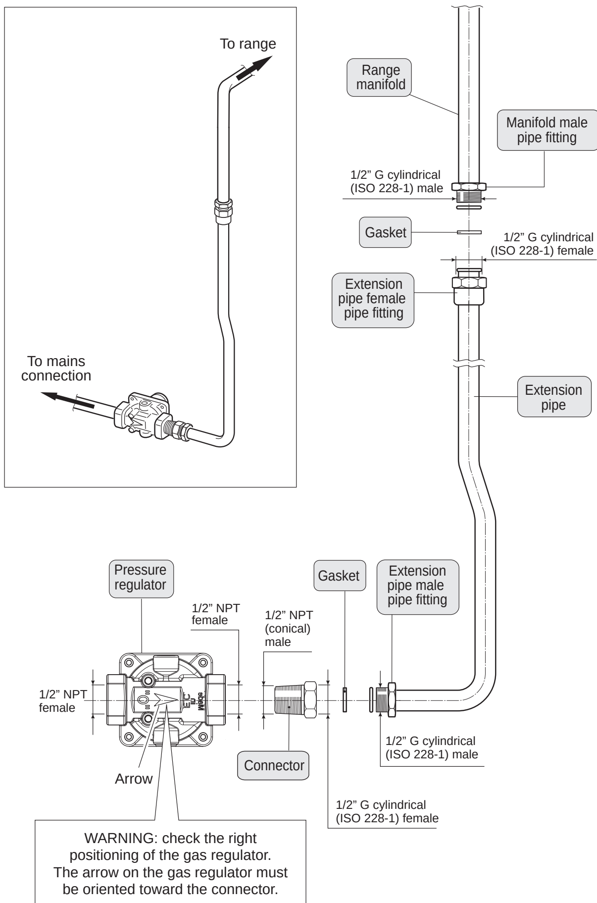
Fig. 2.3
