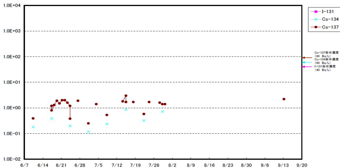
福島第一 南放水口付近 海水放射能濃度(Bq/L)
