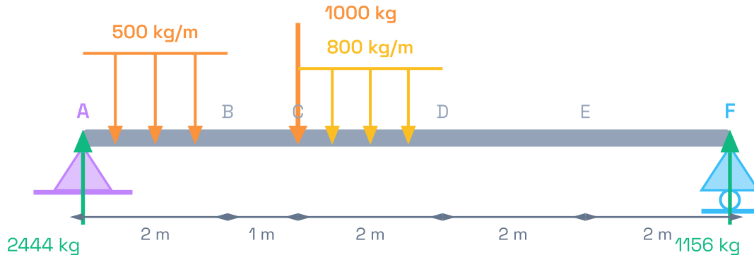
FIGURA — VIGA BIAPOYADA A-F: DOS DISTRIBUCIONES Y CARGA PUNTUAL
