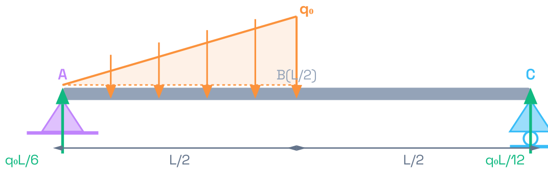
FIGURA — VIGA BIAPOYADA A-C CON CARGA TRIANGULAR EN [0, L/2]
