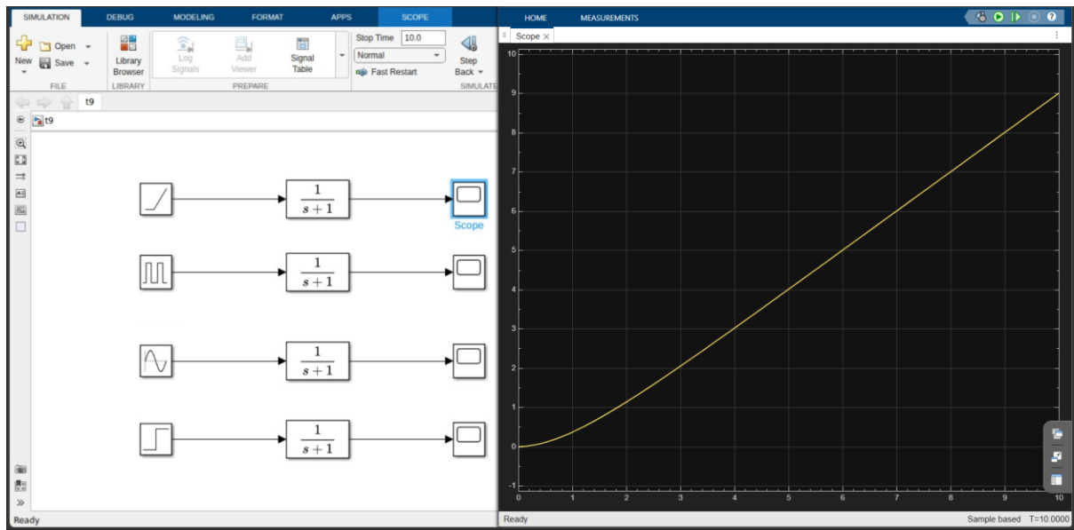
Semnal rampa
