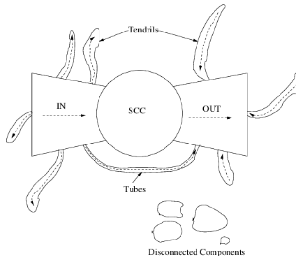
Figura 4.2: Il grafo del web come bowtie
