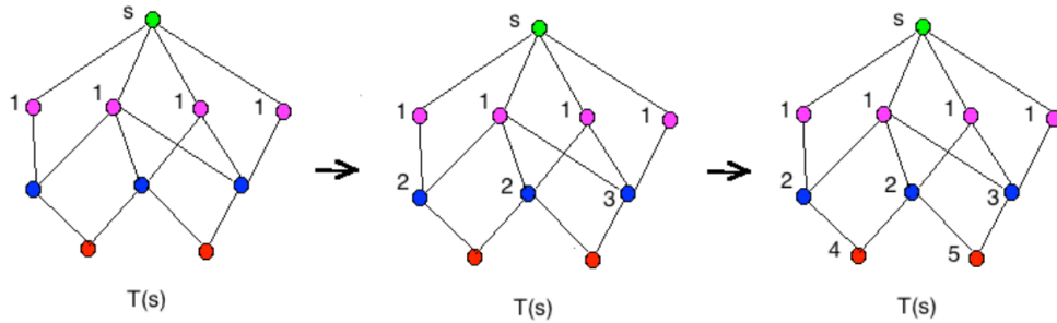
Figura 2.8: Calcolo dei cammini minimi in T(s)
