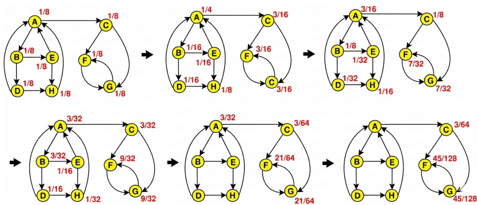
Figura 4.4: Contro esempio in cui il grafo è sconnesso
