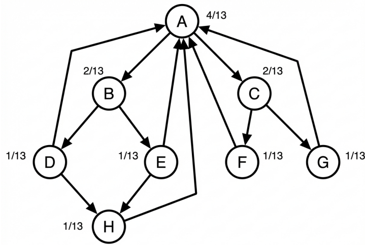
Figura 4.3: Vettore limite a partire da f_i^{(0)} = \frac{1}{8}
