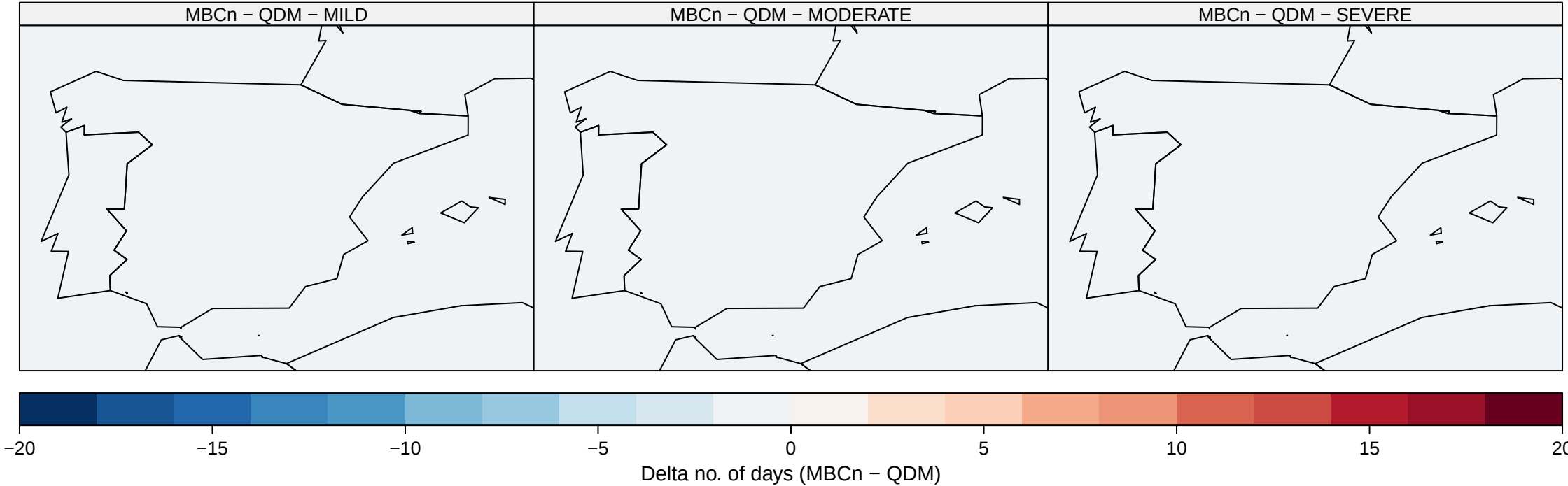
Delta no. of days (MBCn – QDM)
