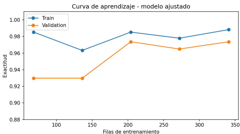
Figura 3. Curva de aprendizaje del modelo ajustado.
