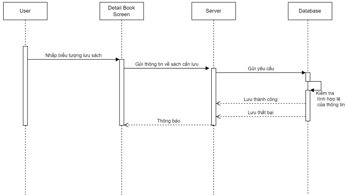
Hình 9.6.2.2. Biểu đồ tuần tự Lưu sách yêu thích
