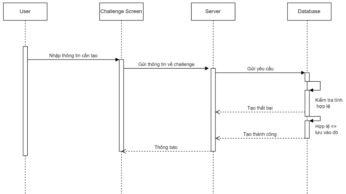
Hình 9.8.2.2. Biểu đồ tuần tự usecase Thêm thử thách
