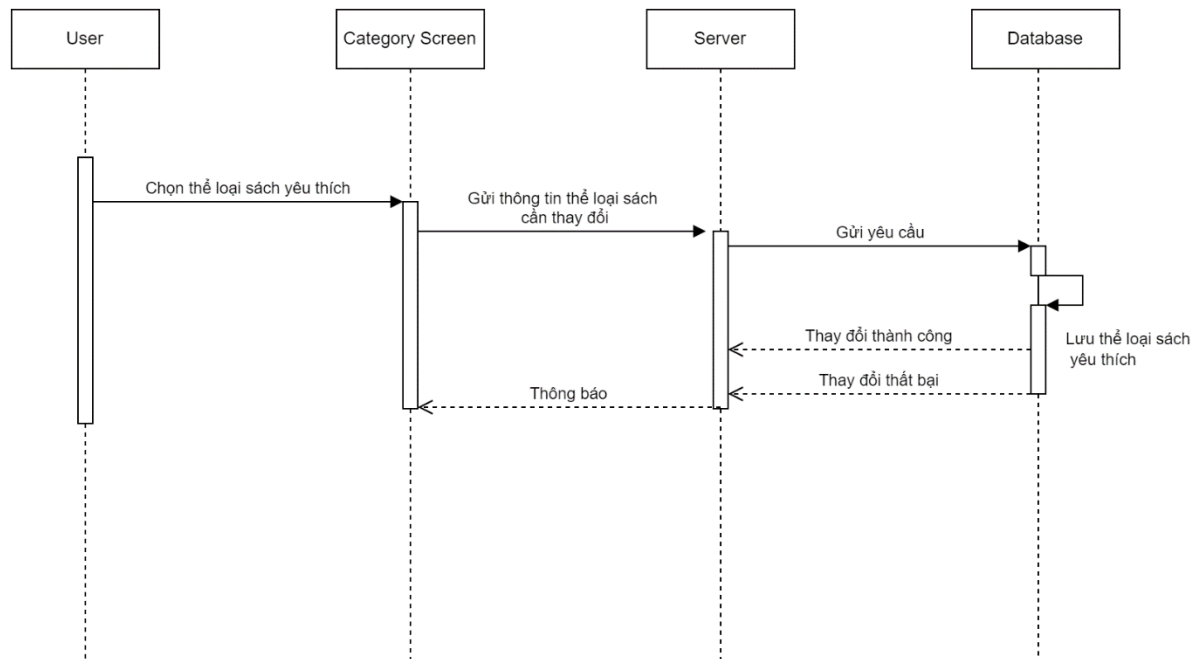
Hình 9.7.3.2. Biểu đồ tuần tự usecase Thay đổi thể loại sách yêu thích
