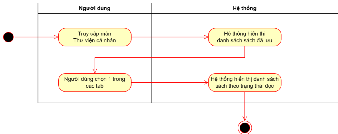
Hình 9.6.1.1. Biểu đồ hoạt động usecase Danh sách sách thư viện
