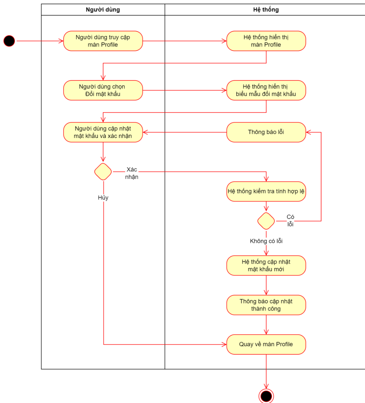
Hình 9.7.2.1. Biểu đồ hoạt động usecase Đổi mật khẩu
