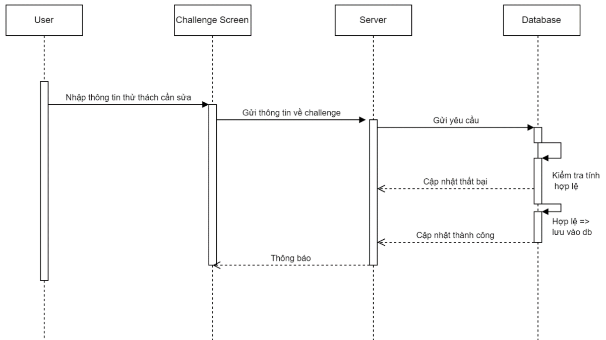
Hình 9.8.3.3. Biểu đồ tuần tự usecase Sửa thử thách
