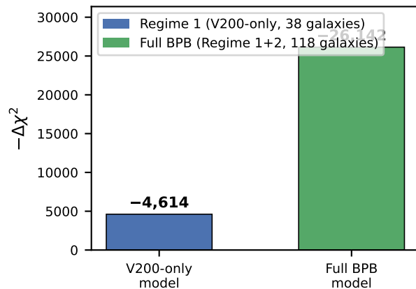
(d) \Delta\chi^2 summary
