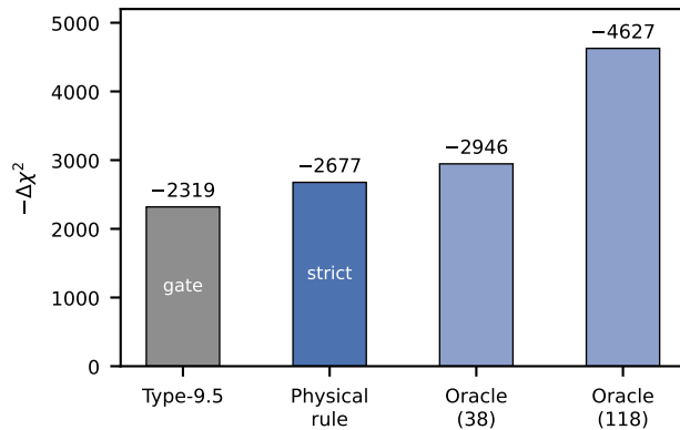
(d) \Delta\chi^2 summary
