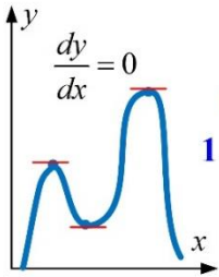
求极值
