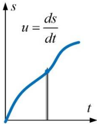
瞬时速度
