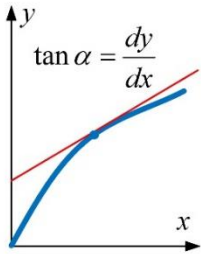
求切线
