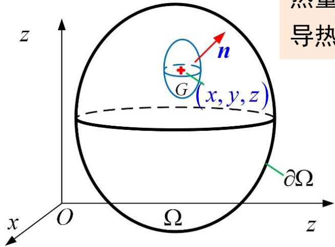
导热体传热分析
