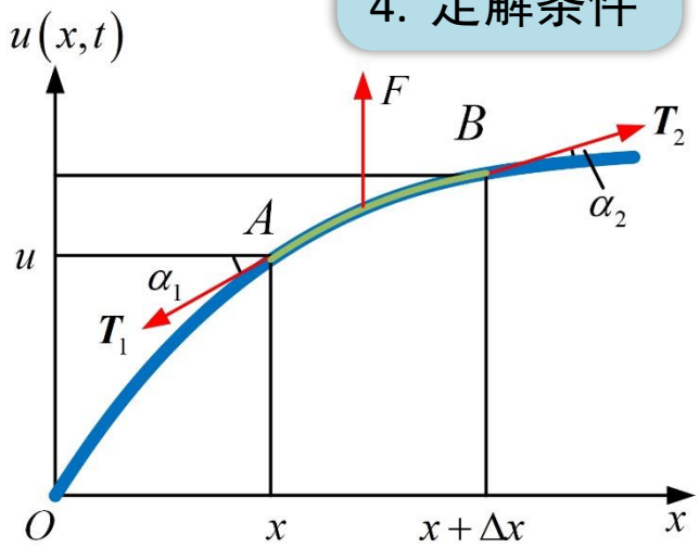
弦振动受力分析
