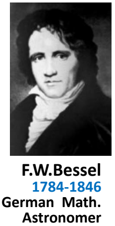
r 阶Bessel函数
