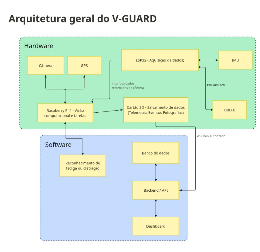
Figura 3: Arquitetura geral do V-GUARD.
