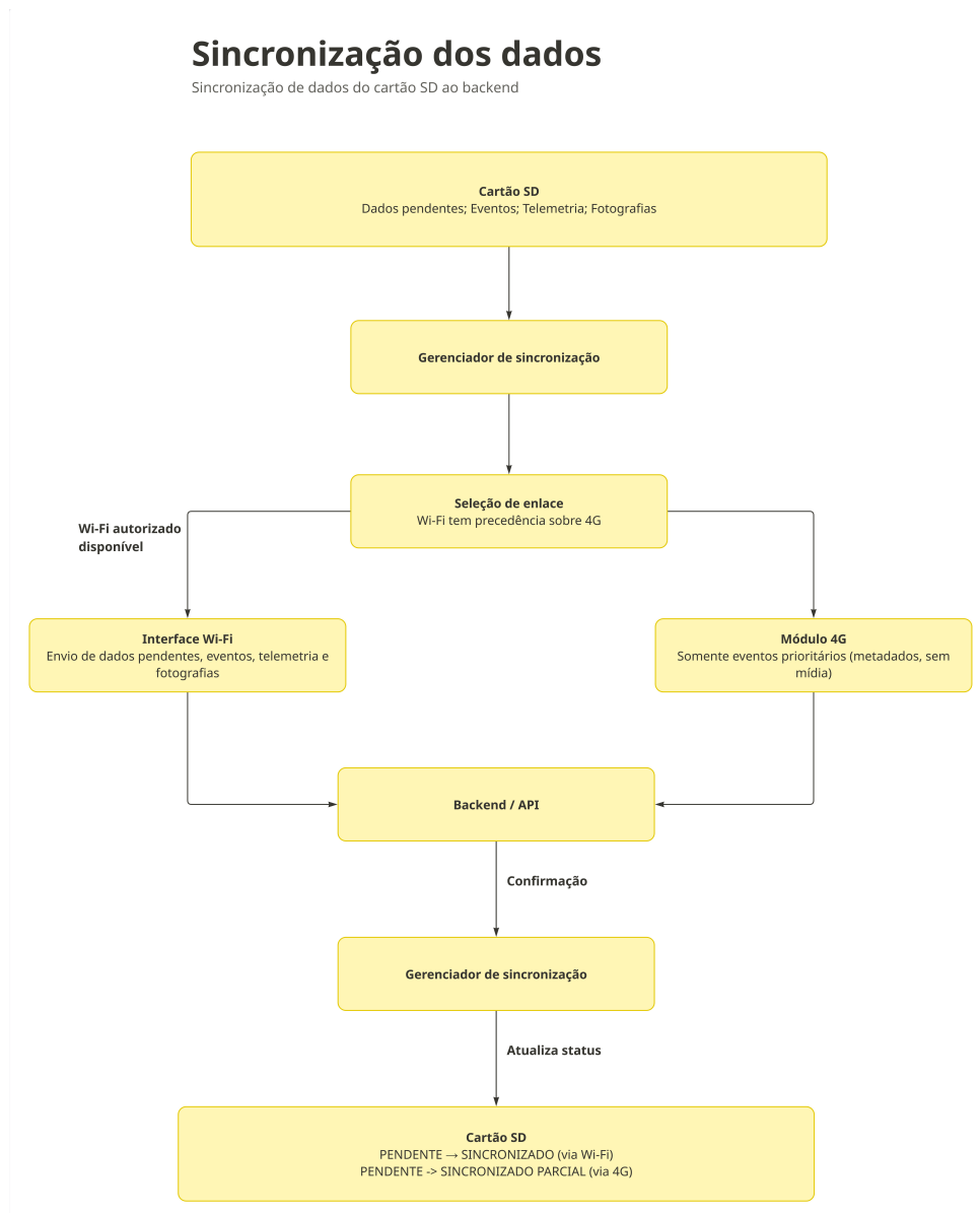
Figura 5: Sincronização dos dados.
