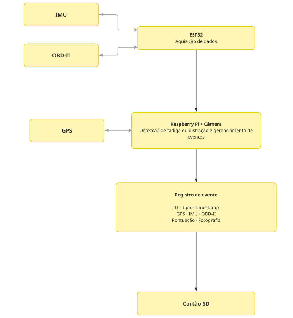
Figura 4: Gerenciamento de eventos.
