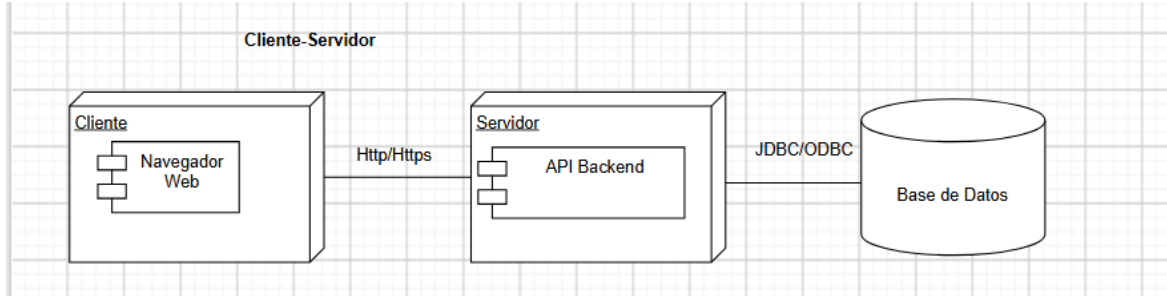
Fig. 1 Arquitectura Cliente-Servidor
