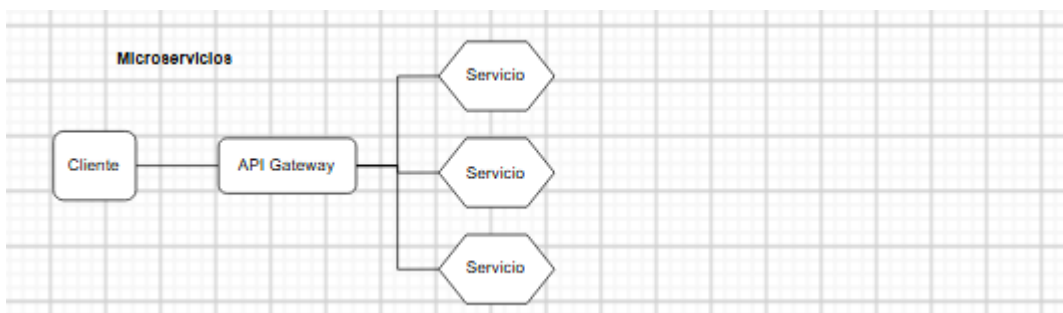
Fig. 4 Arquitectura Microservicio
